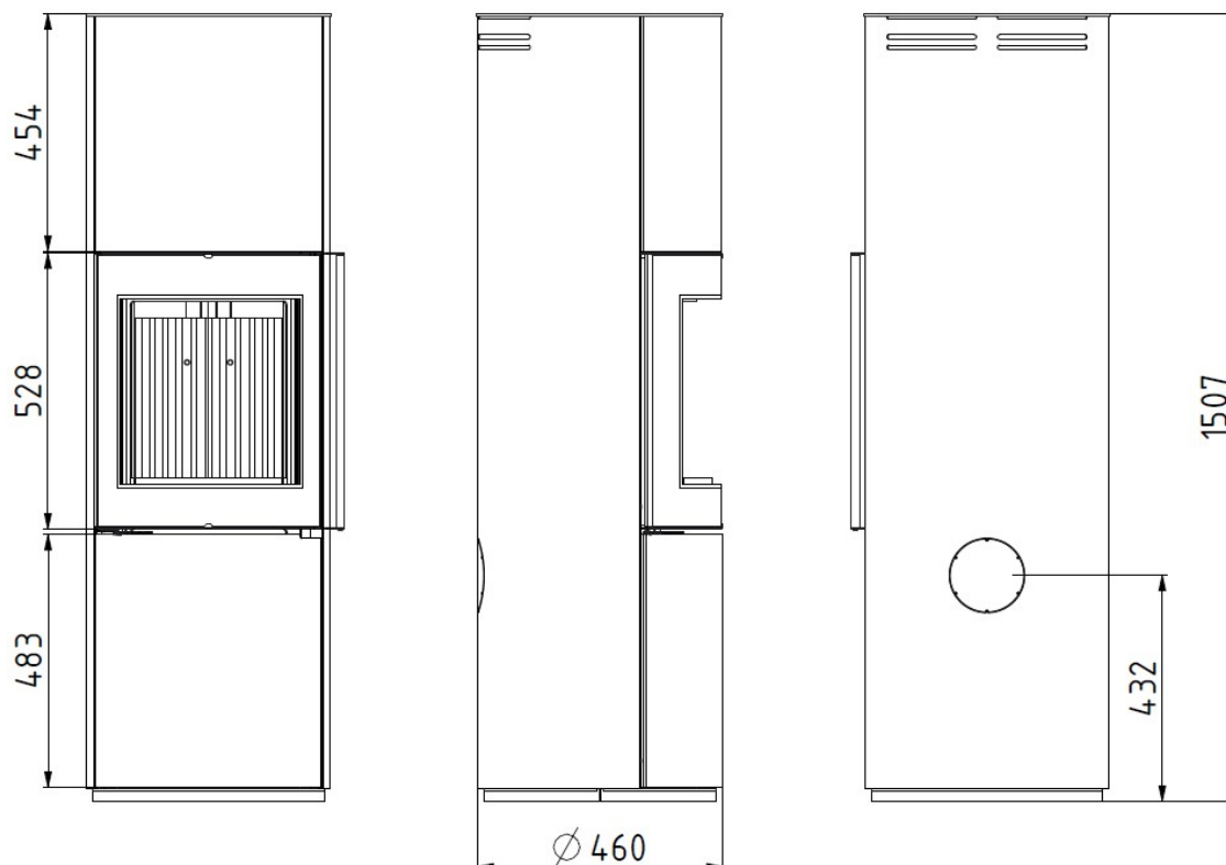
Slika 2: Dimenzije peči Vintgar150A
